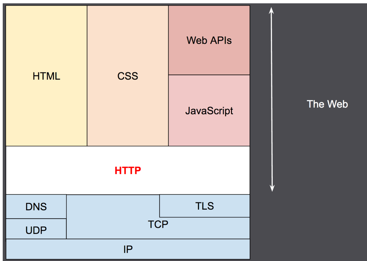
Figura 2: Capas HTTP
