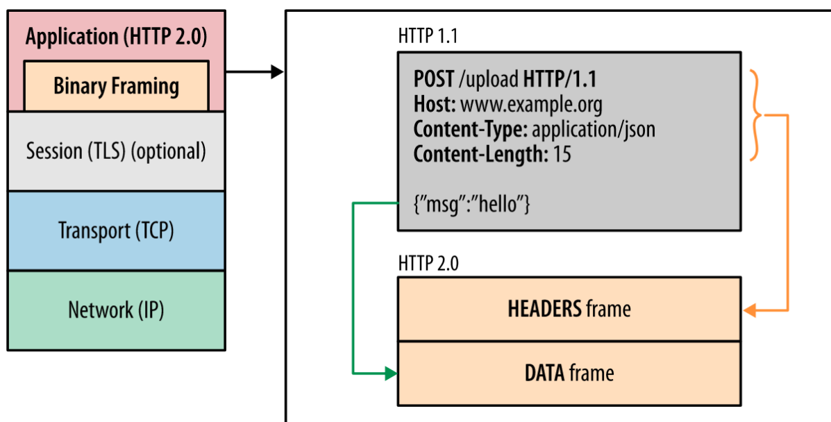
Figura 11: Capa de entramado binario de HTTP/2
